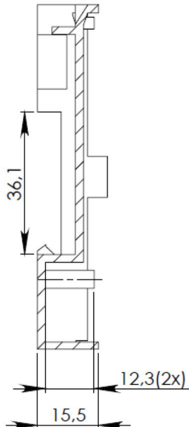
PRZEKRÓJ B-B
