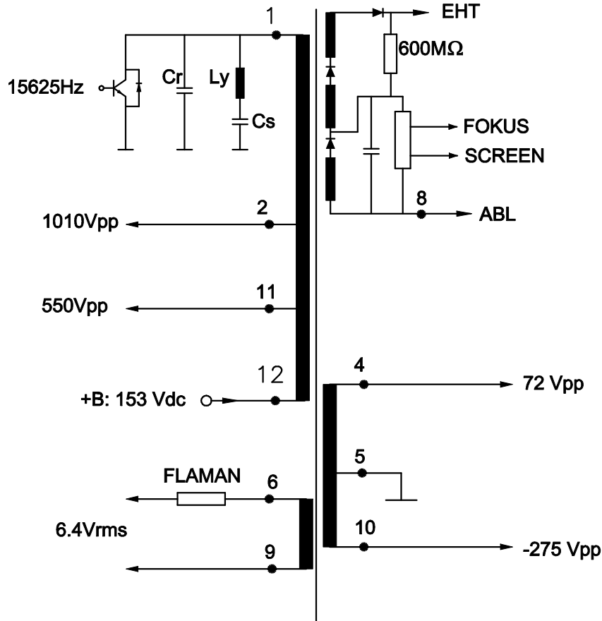
Elektriksel Diagram
