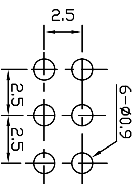
P.C.B HOLE DETAIL
