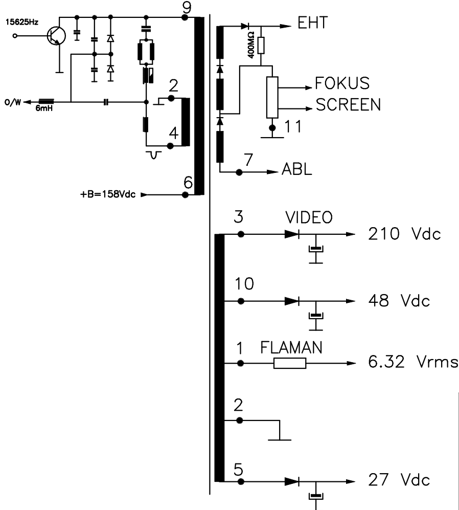
Elektriksel Diagram
