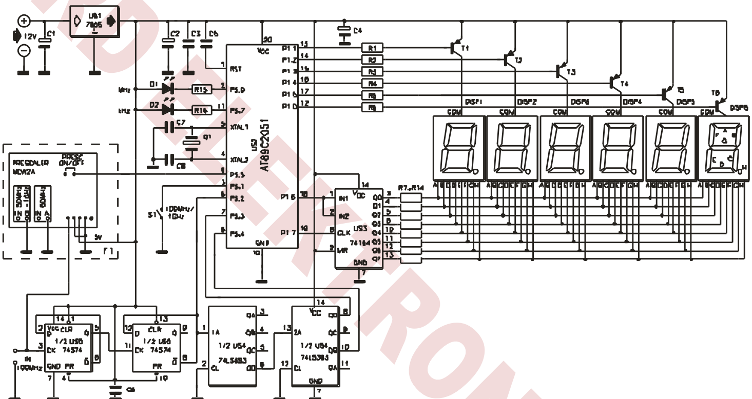
Rysunek 2. Schemat ideowy płytki bazowej
