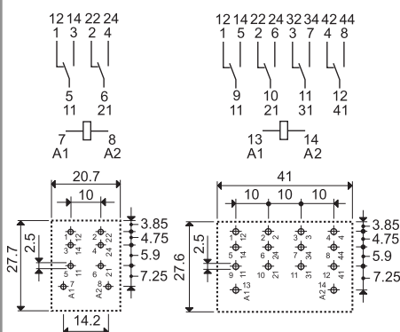
56.42 56.44 pohled ze strany vývodů
