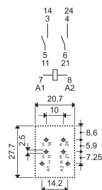
56.42-0300 pohled ze strany vývodů
